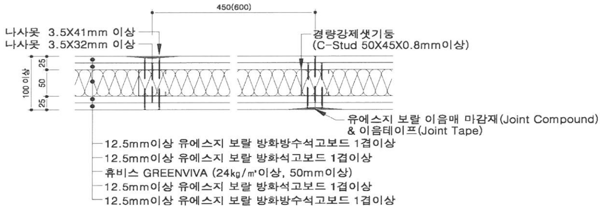
평면 상세도
