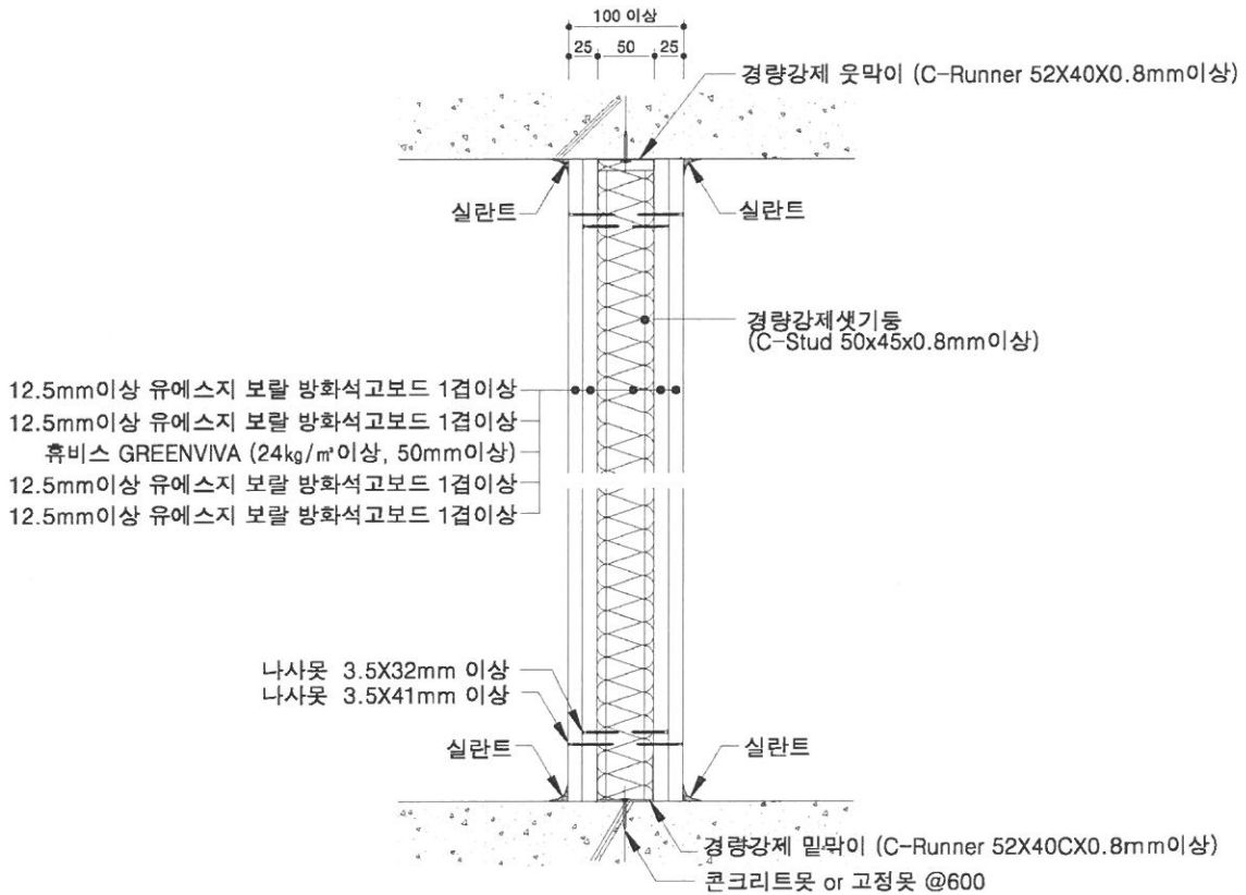
[수직단면 상세도]
