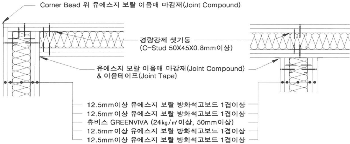
[ “┌” / “T” 접합부위 상세도 ]
