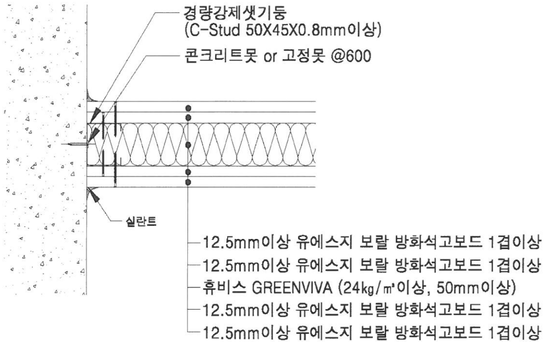
[ 벽 접합 상세도 ]
