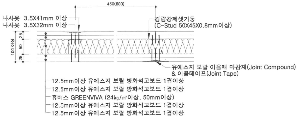
[수평단면 상세도]
